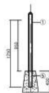
측면도
