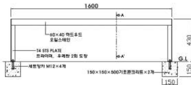
정면도
