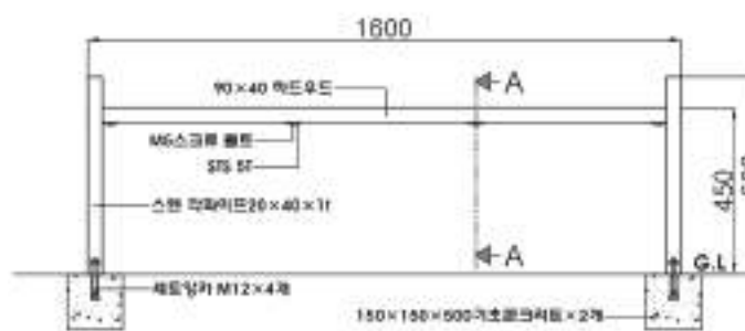
정면도
