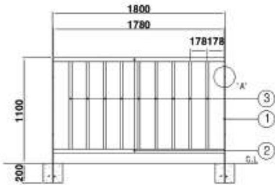
정면도
