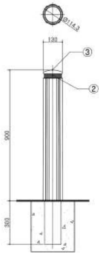
측면도
