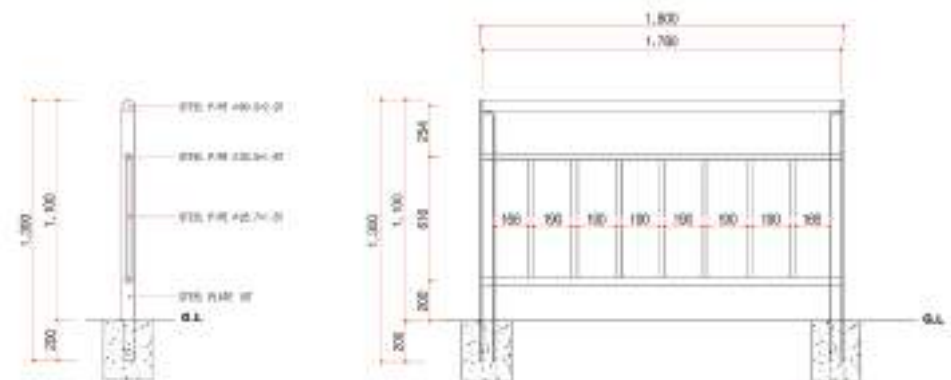
단면도
