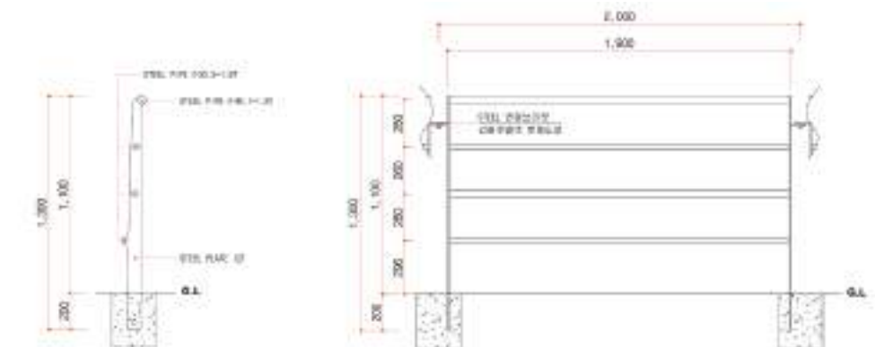
단면도
