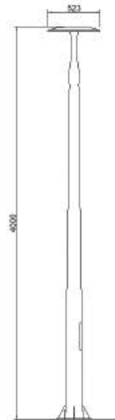
측면도
