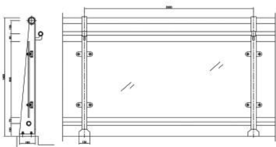
단면도
