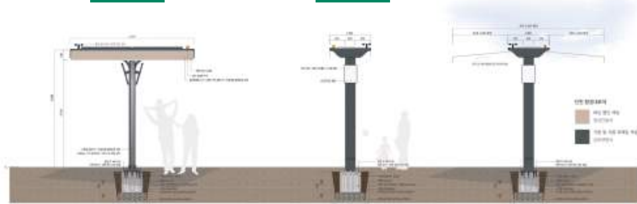
정면/배면도
