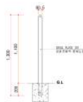
측면도
