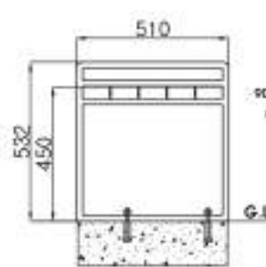
우측면도
