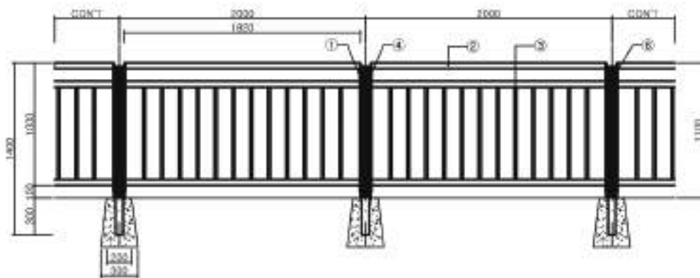
전개도
