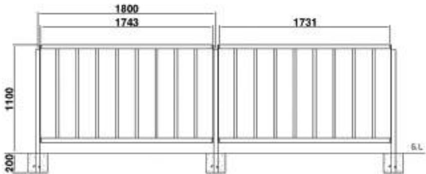
전개도
