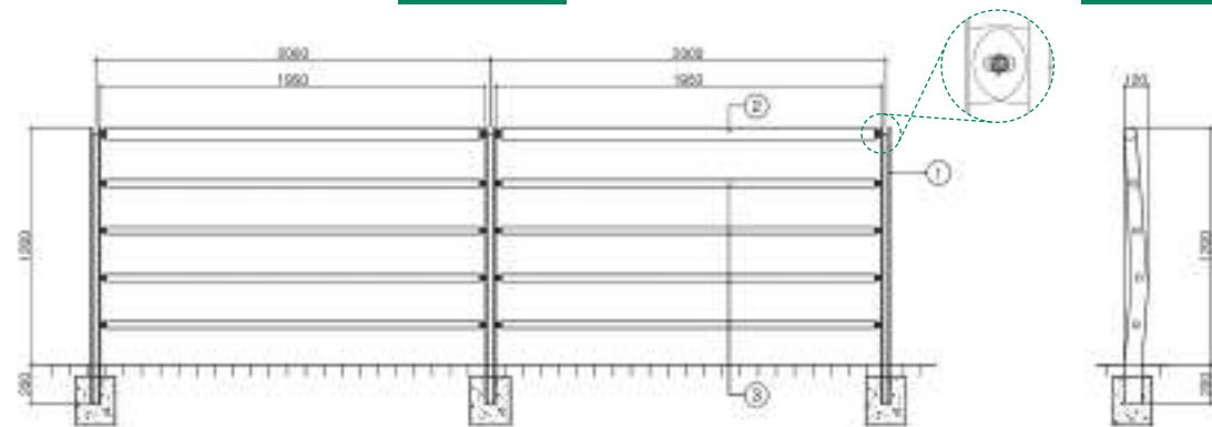
전개도
