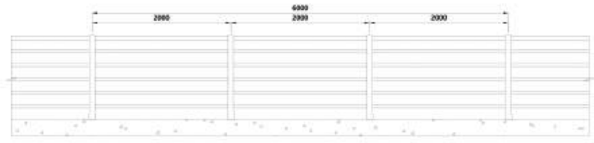
전개도
