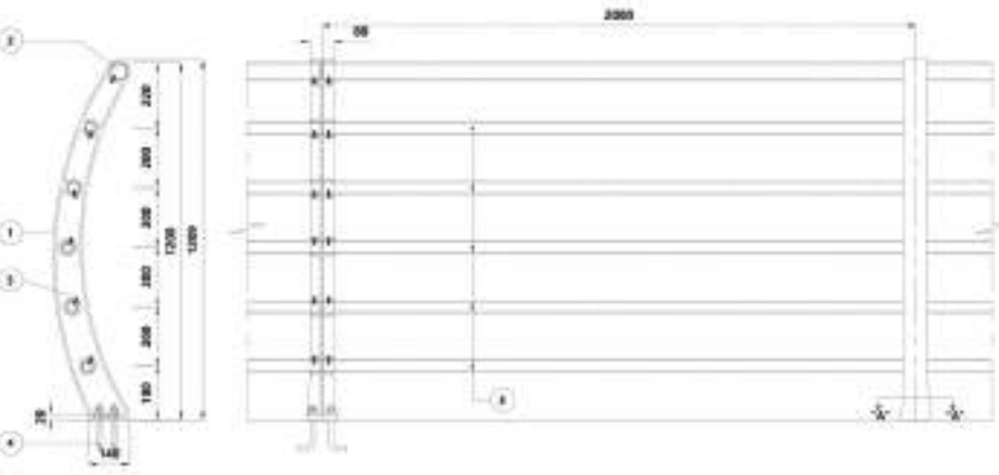
단면도
