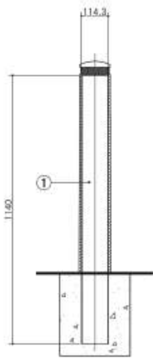
정면도
